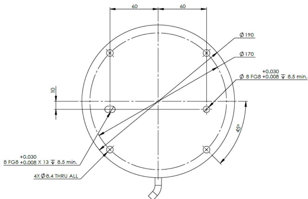
1.1: 机器人基座的底部视图
