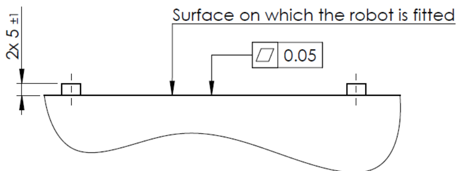
1.2: 机器人基座安装板
